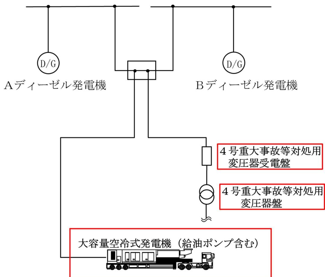
【電源系統図】
