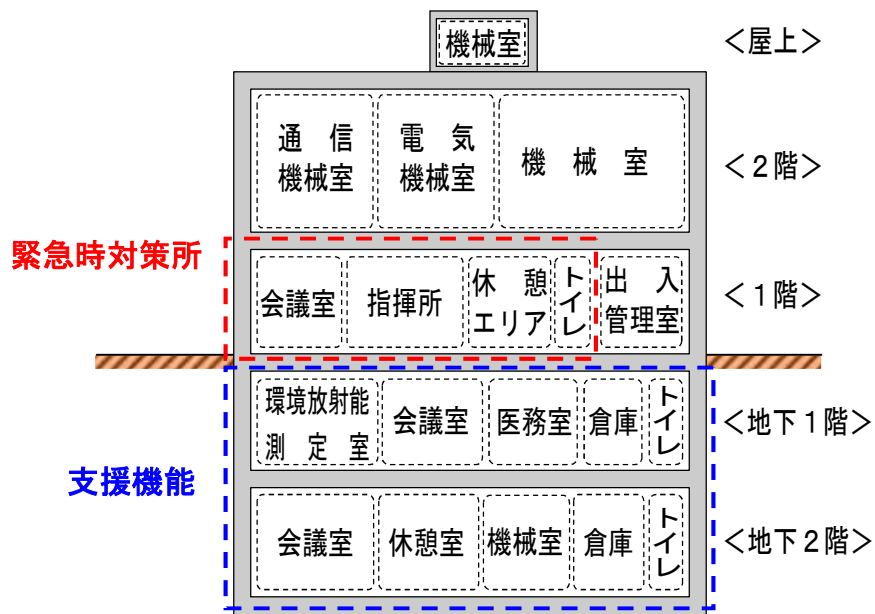
【 断面図 】
