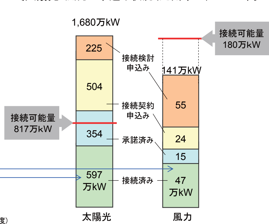
〔太陽光・風力の申込み状況(九州本土)2016.3末〕
