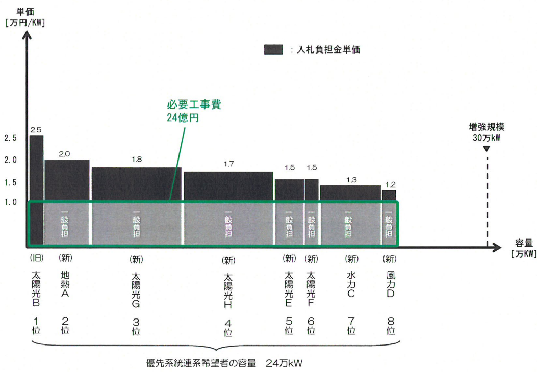
〔①入札対象工事（220/110kV 変圧器増強工事）〕
