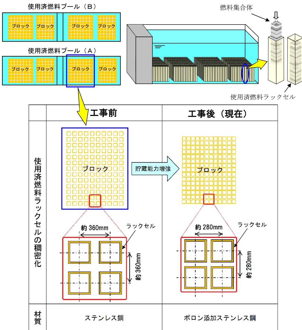
【使用済燃料プール貯蔵能力増強概要図】
