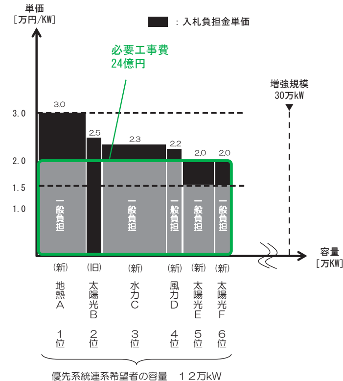
〔①入札対象工事 (220/110kV 変圧器増強工事) 〕
