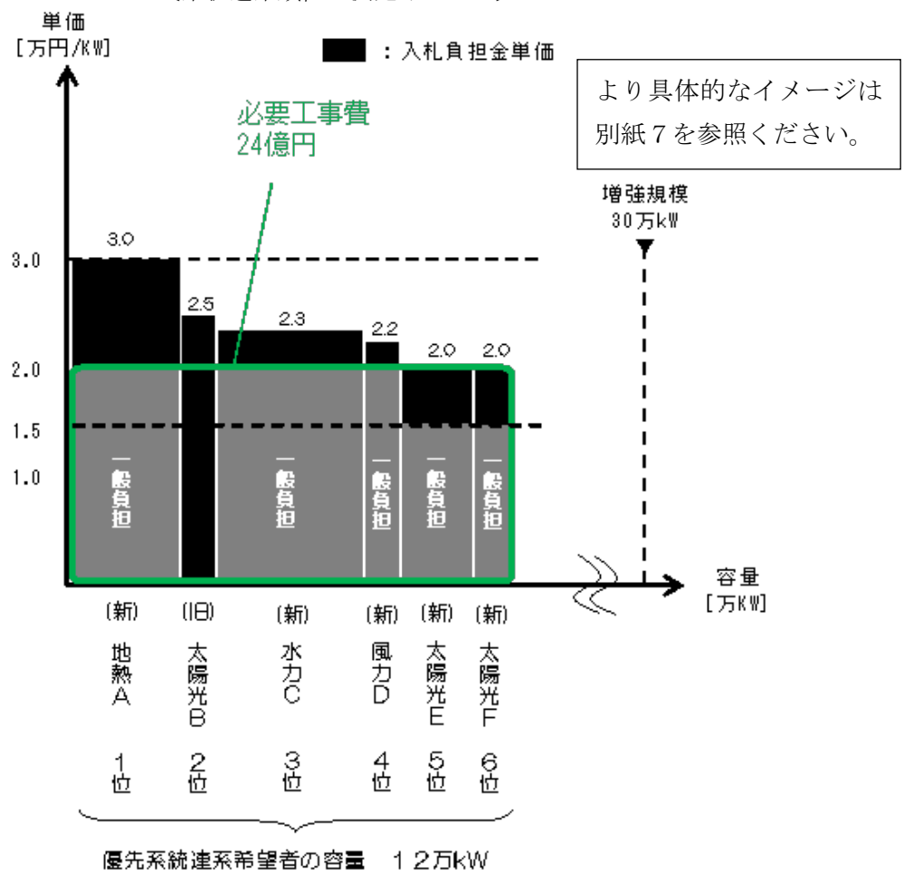
[系統連系順位の決定イメージ]
