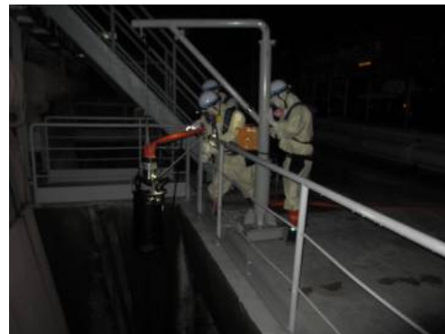
取水用水中ポンプの現場設置訓練
