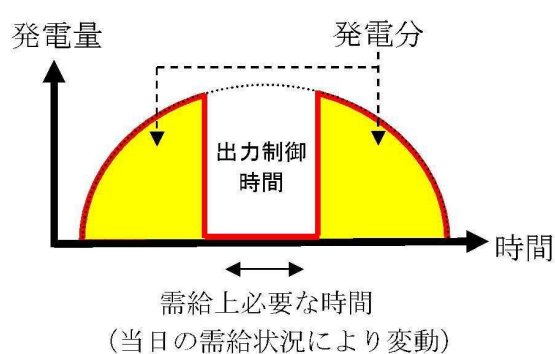
【オンライン発電所の出力制御イメージ】
