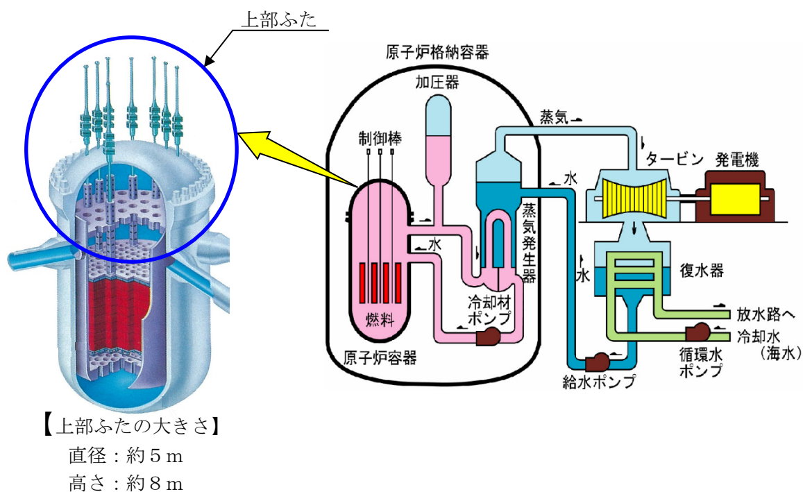
<原子炉容器上部ふた概要図>
