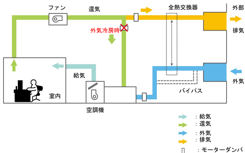
代表的なダクト系統図
