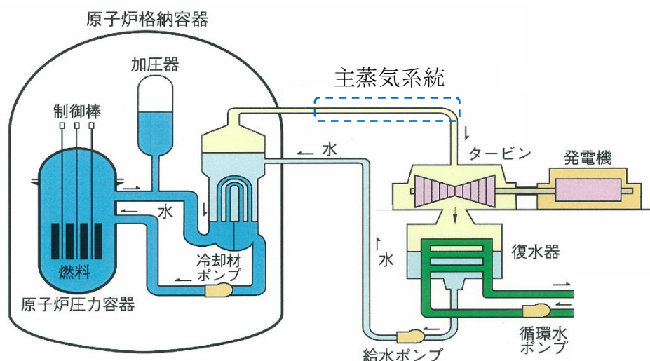
【発電所概要図】
