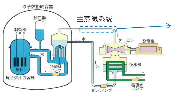
【発電所概要図】
