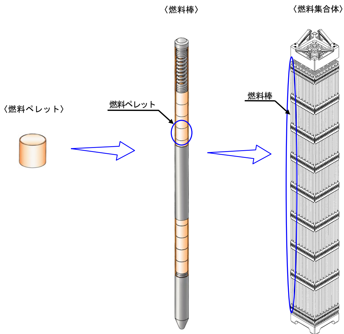
【燃料集合体概要図】
