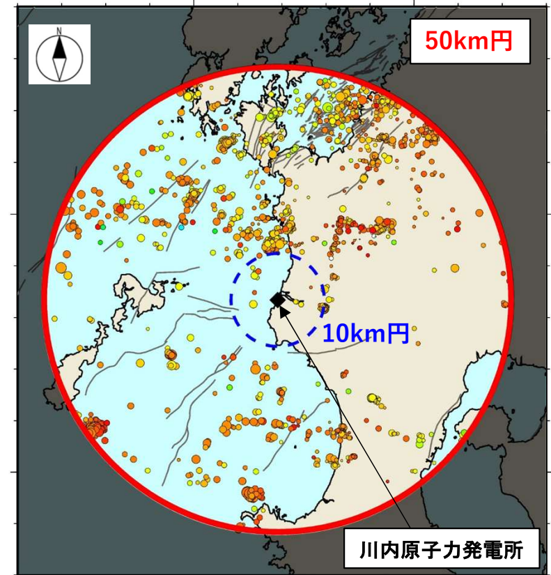
2024年度の震央分布図 (2024年4月～2025年3月)
