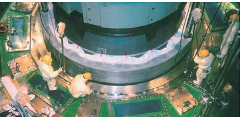
原子炉容器蓋取外し作業
