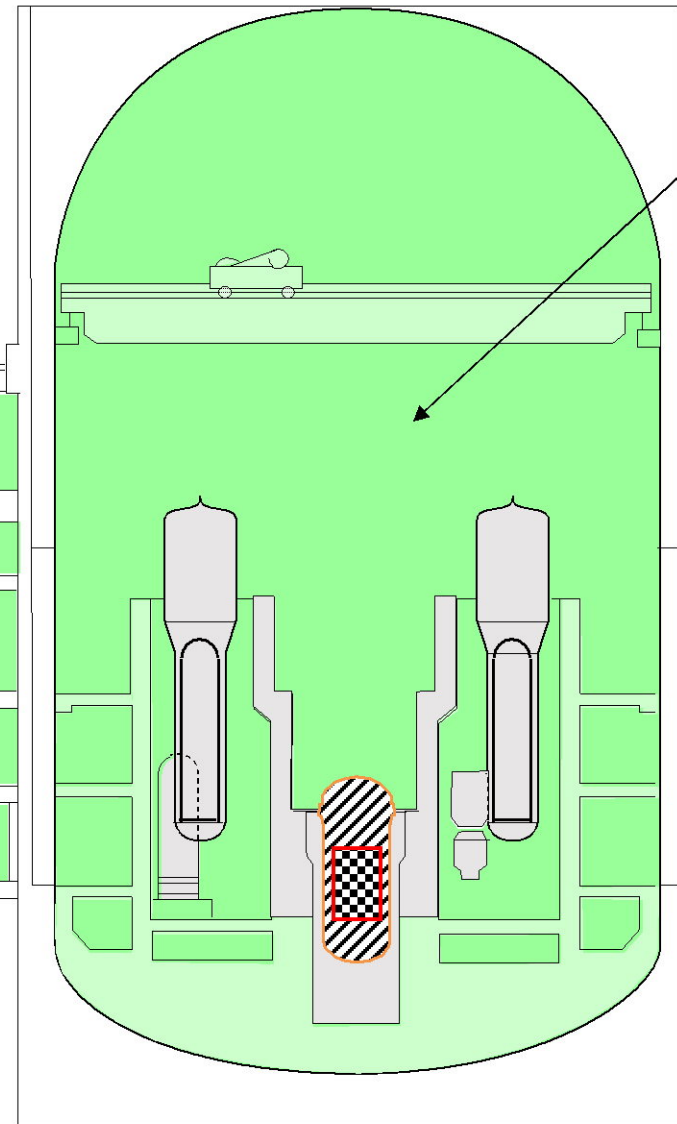
第 5.3.1 図 主な廃止措置対象施設の推定汚染分布
