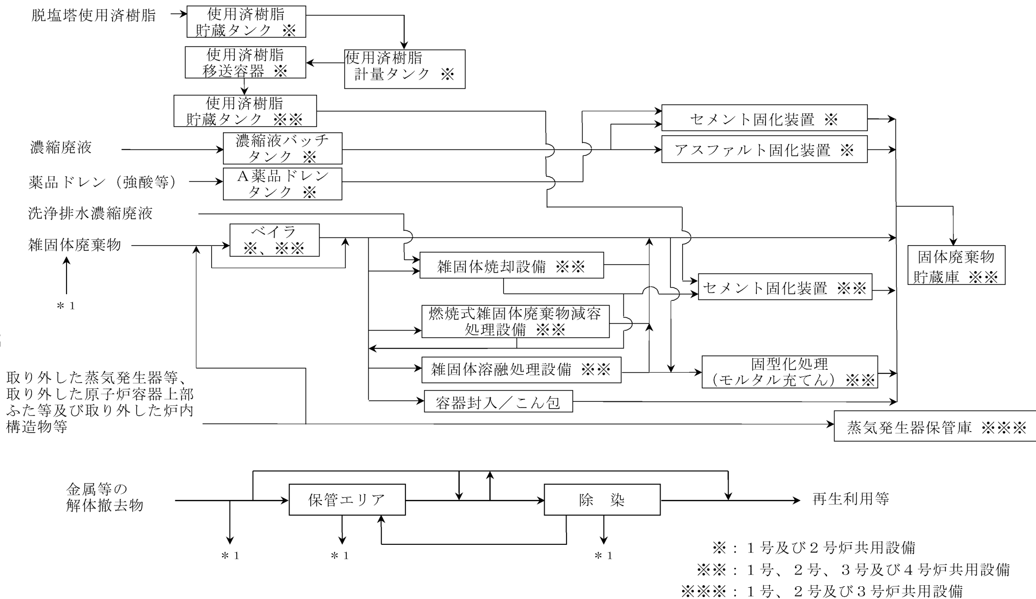
第 10.7 図 原子炉周辺設備等解体撤去期間中の放射性固体廃棄物の処理フロー
