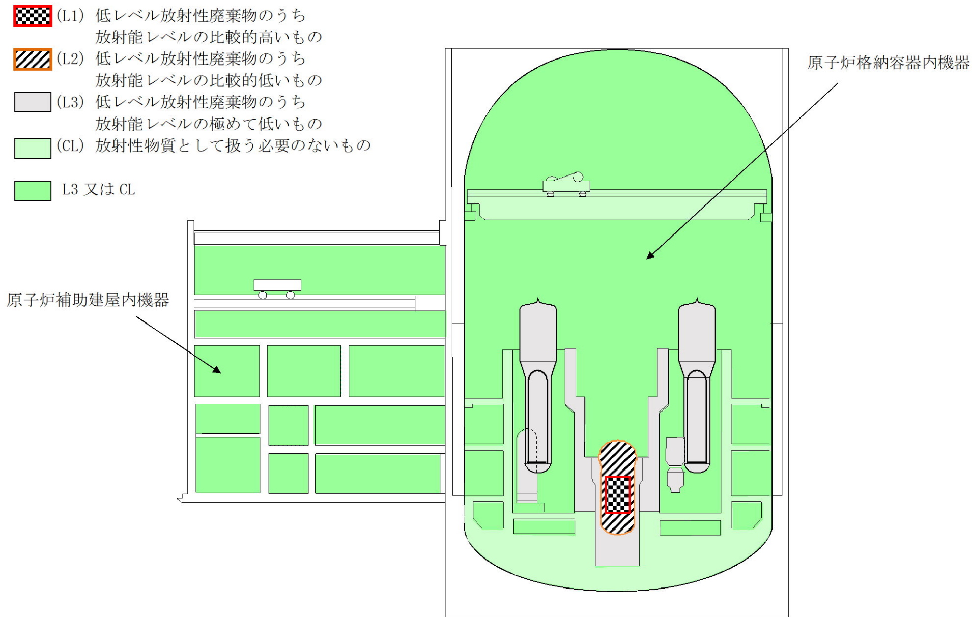
第 9.1 図 汚染の推定分布図
