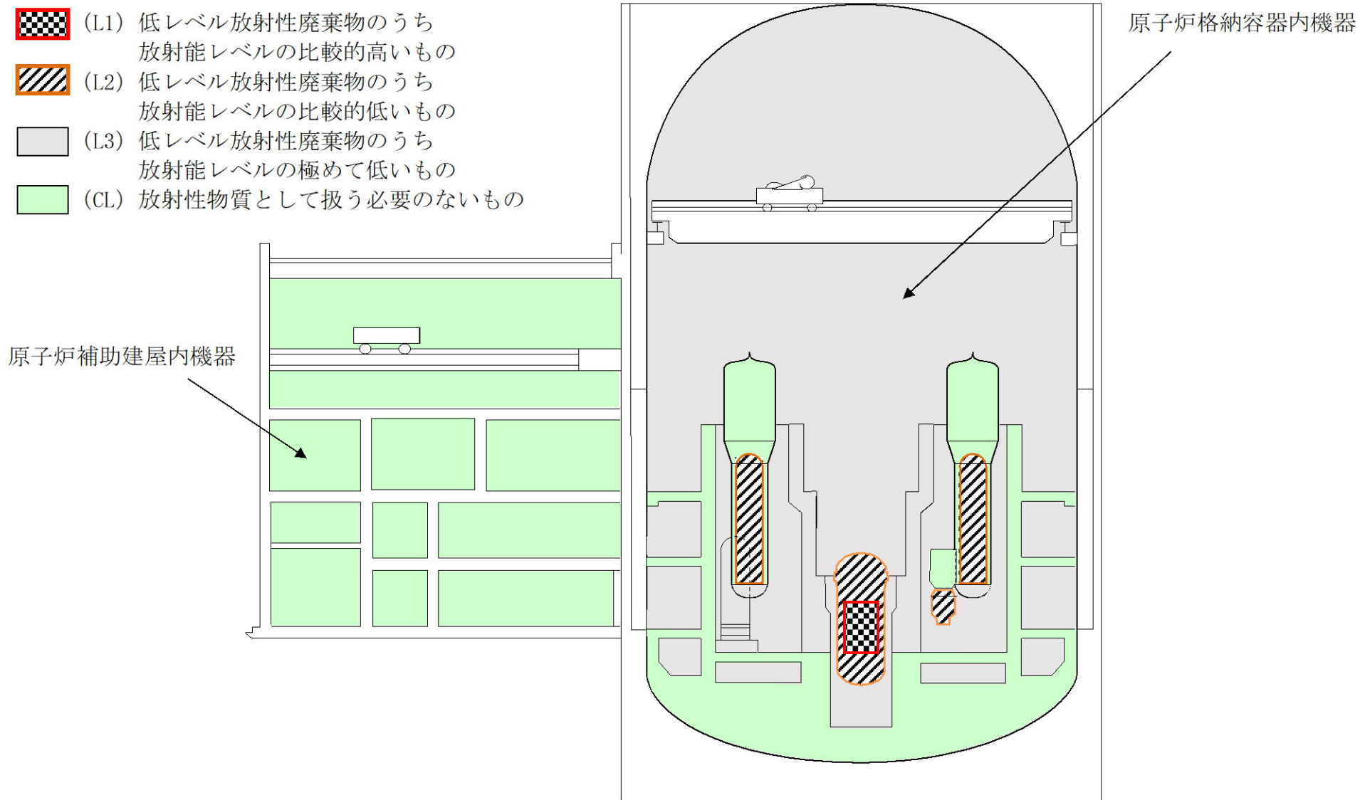
第 4.3 図 主な廃止措置対象施設の推定汚染分布（初回申請）
