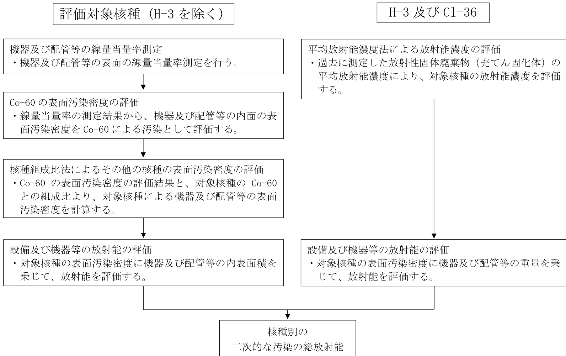
第 5.2.2 図 二次的な汚染の評価方法
