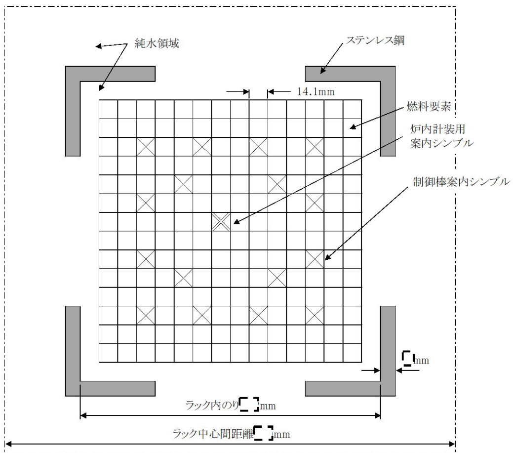
第3図 使用済燃料ピット水大規模漏えい時の未臨界性評価の計算体系 (水平方向、燃料体部拡大)
