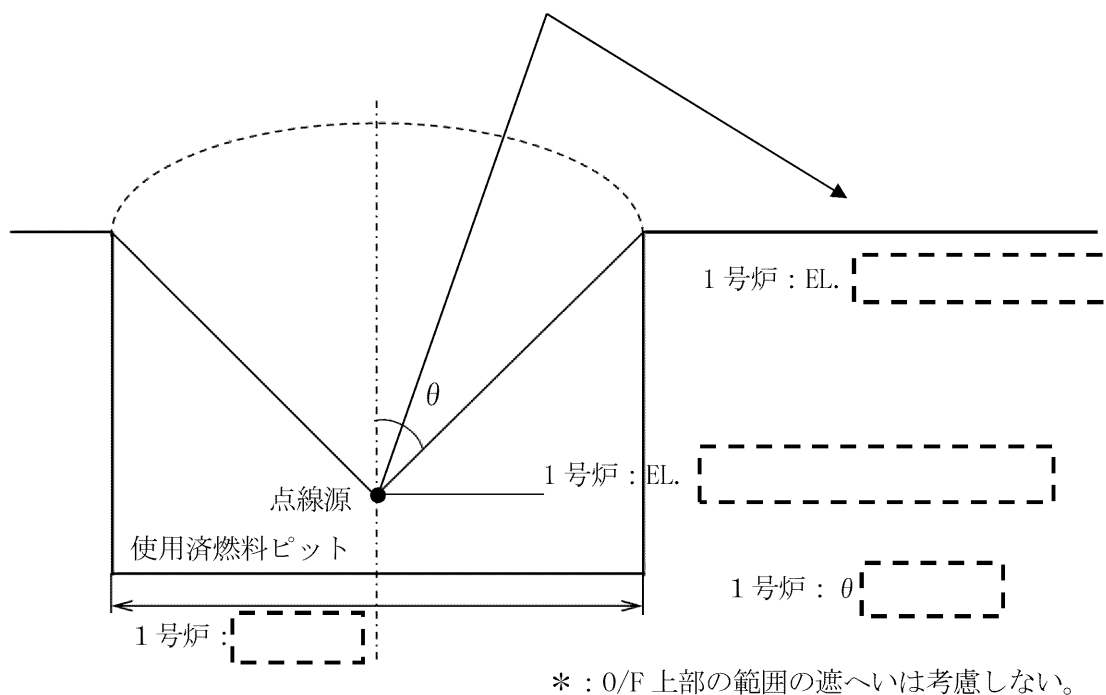
図 1 評価モデル
