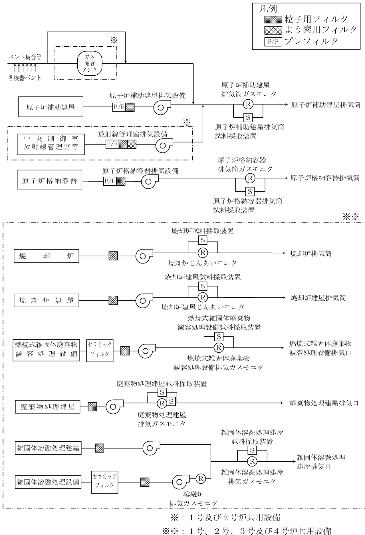
第 10.1 図 解体工事準備期間中の放射性気体廃棄物の処理処分フロー
