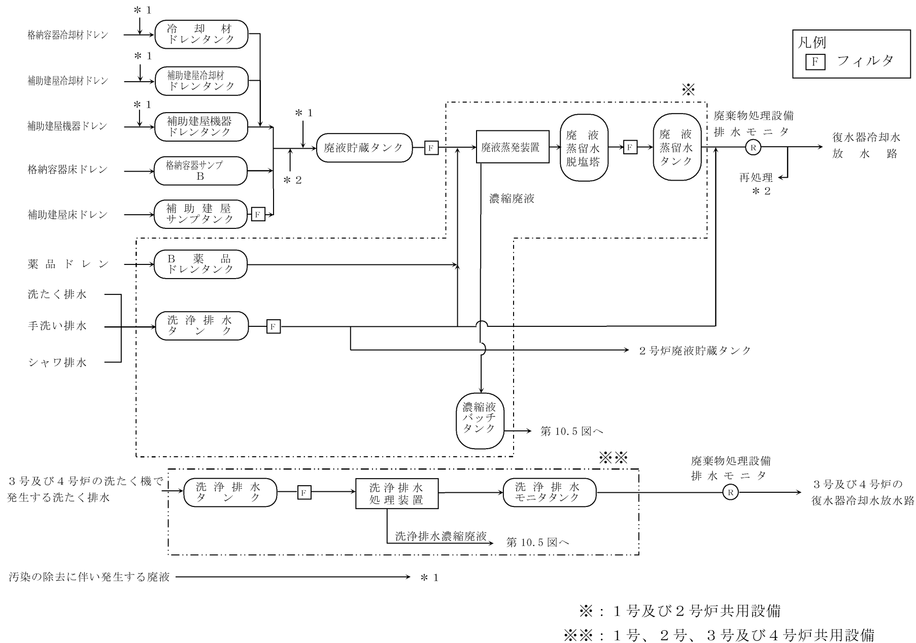
第 10.3 図 解体工事準備期間中の放射性液体廃棄物の処理処分フロー
