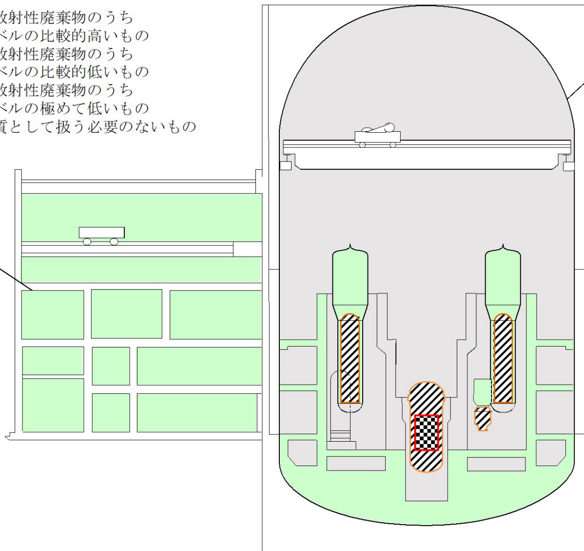
第 5.1.1 図 主な廃止措置対象施設の推定汚染分布（初回申請）
