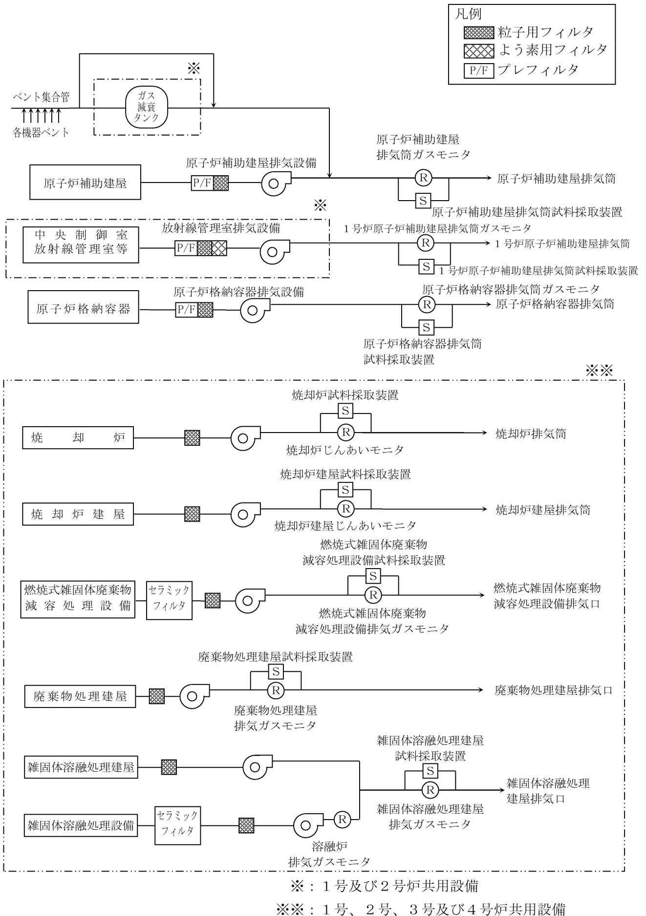
第 10.1 図 解体工事準備期間中の放射性気体廃棄物の処理処分フロー
