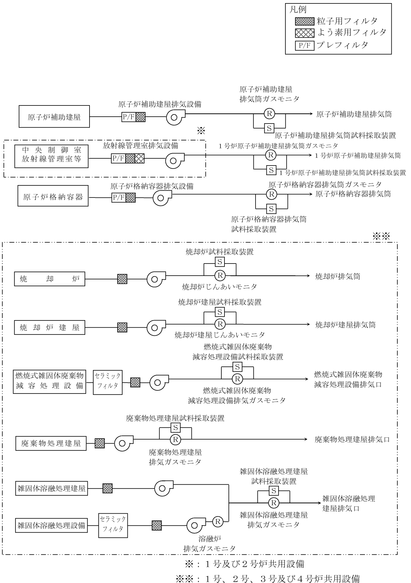
第 10.2 図 原子炉周辺設備等解体撤去期間中の放射性気体廃棄物の処理処分フロー
