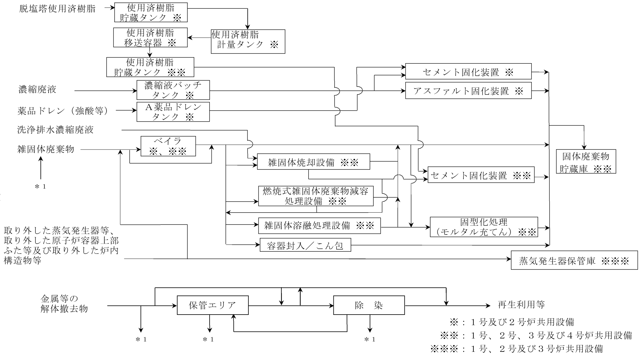
第 10.7 図 原子炉周辺設備等解体撤去期間中の放射性固体廃棄物の処理フロー
