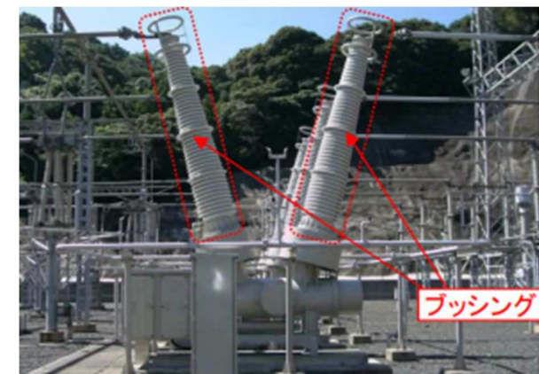
[遮断器外観]
