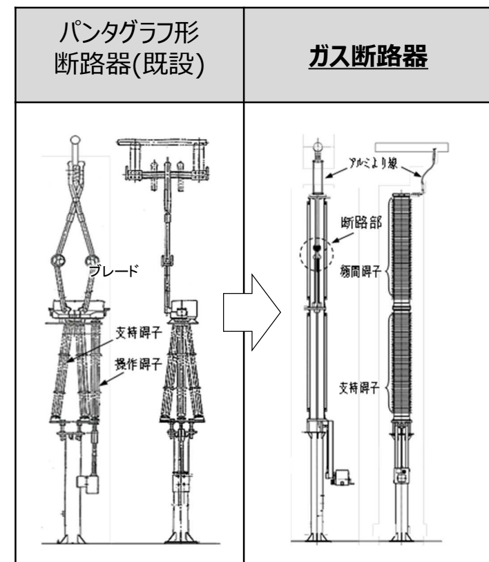
新たに導入する断路器 の構造図
